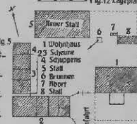
Fig. 12 Lageplan
