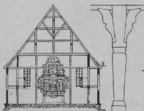
Fig. 7 Querschnitt
