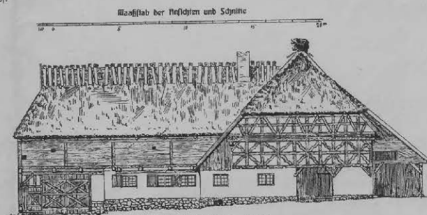
Fig. 5 Ansicht des Gehöftes von Osten
