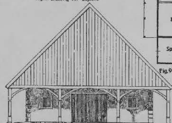
Fig. 13 Hofseit. des Stallalles
