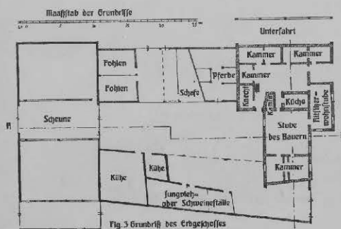
Fig. 3 Grundriß des Erdgeschosses
