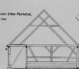
Fig. 5 Querschnitt durch die Scheune Fig. 9
