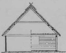
Fig. 1 Schnitt durch die Scheune
