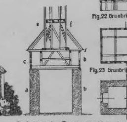
Fig. 21 Schnitt des Thurmes
