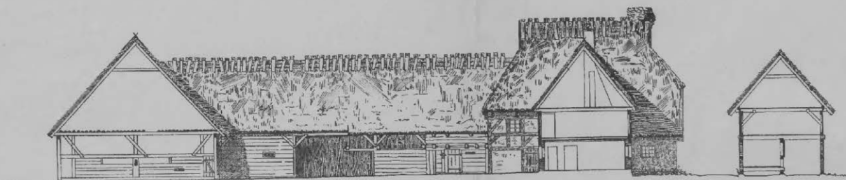
Fig. 2 Längsschnitt A—B durch das Gehöft
