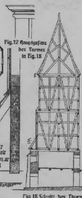
Fig. 18 Schnitt des Turmes
