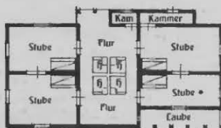
Abb. 31. Fig. 1. Insthaus in Kobbelbude, Kreis Fischhausen. Fig. 2. Insthaus in Kobbelbude, Kreis Fischhausen. Fig. 3. Fischerhaus für 4 Familien in Gllge, Kreis Cahlau.
