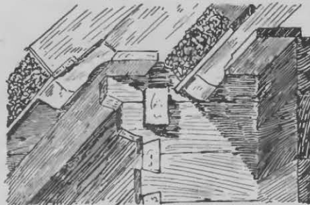
Fig. 2. Gehrfaßecklösung in Gilge, Kreis Labiau, Haus Lepkojls.
