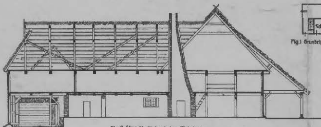
Fig. 1-5 Gehöft des Besizers Thron
