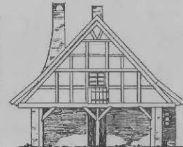
Fig. 12 Giebelansicht zu Fig. 5
