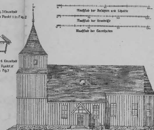
Fig. 5 Seitenansicht
