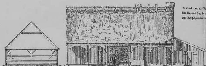
Fig. 4 Schnitt durch die Scheune und Hofseit. der Scheune Fig. 9
