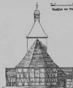
Fig. 2 Ansicht der Offseite
