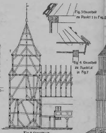
Fig. 2 Längsschnitt
