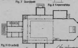
Fig. 11 Grundriß
