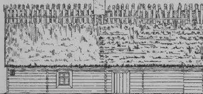
Fig. 5 Ansicht gegen Wohnhaus und Stall
