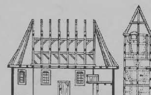
Fig. 5 Längsschnitt
