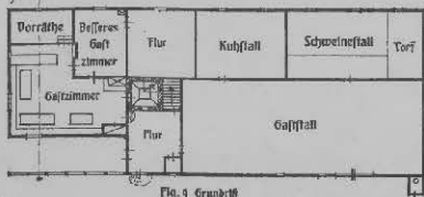
Fig. 4 Grundriß
