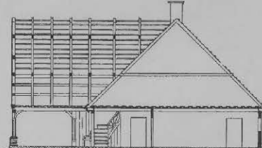
Fig. 3 Querschnitt durch das Wohnhaus
