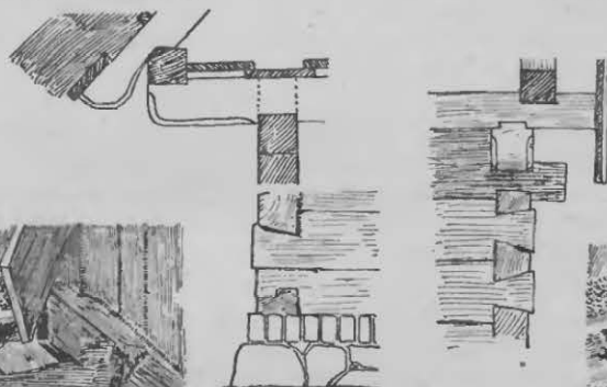
Fig. 3 u. 4. Gehrfaßeckverband und Sparrenauflagerung in Timber, Kreis Labiau.
