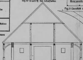
Fig. 14 Querschnitt des Stallalles
