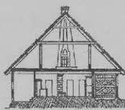
Fig. 2 Schnitt A-B zu Fig. 4
