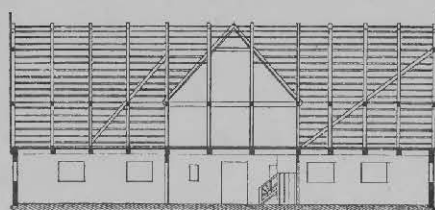
Fig. 1 Längsschnitt durch das Wohnhaus
